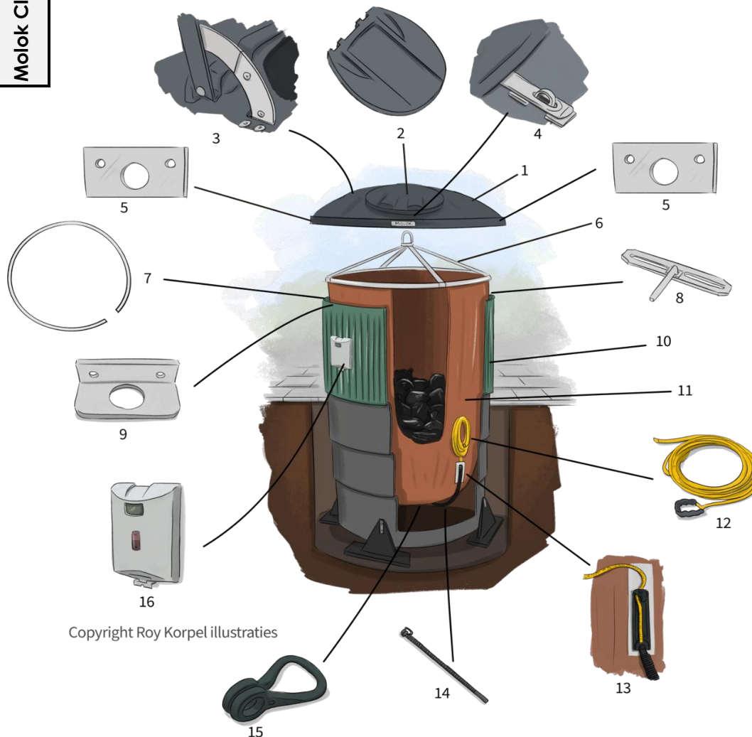
Deksel scharnier 3m3, 5m3 1300 en 800 liter
